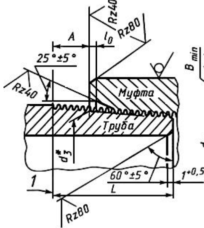
Соединение, свинченное вручную
