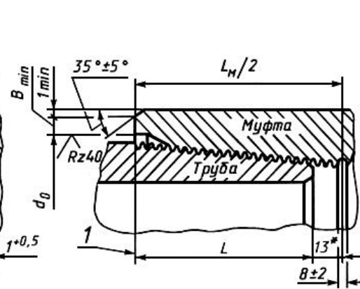
Соединение, свинченное на станке
